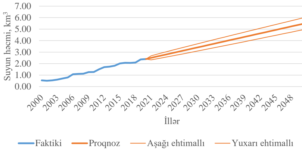
Şəkil 5. Yeraltı su mənbələrindən götürülən suyun həcmnin dəyişməsinin proqnozlaşdırılması
