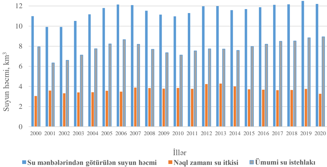
Şəkil 11. Təbii mənbələrdən götürülən və istifadə olunan şirin suyun dəyişməsi
