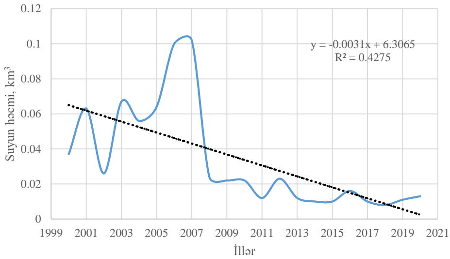
Şəkil 8. Emal sənayesi tərəfindən götürülən suyun həcmnin dəyişməsi
