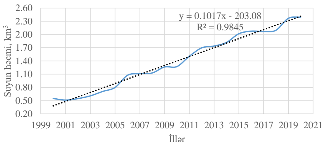
Şəkil 4. Yeraltı su mənbələrindən götürülən suyun həcmnin dəyişməsi
